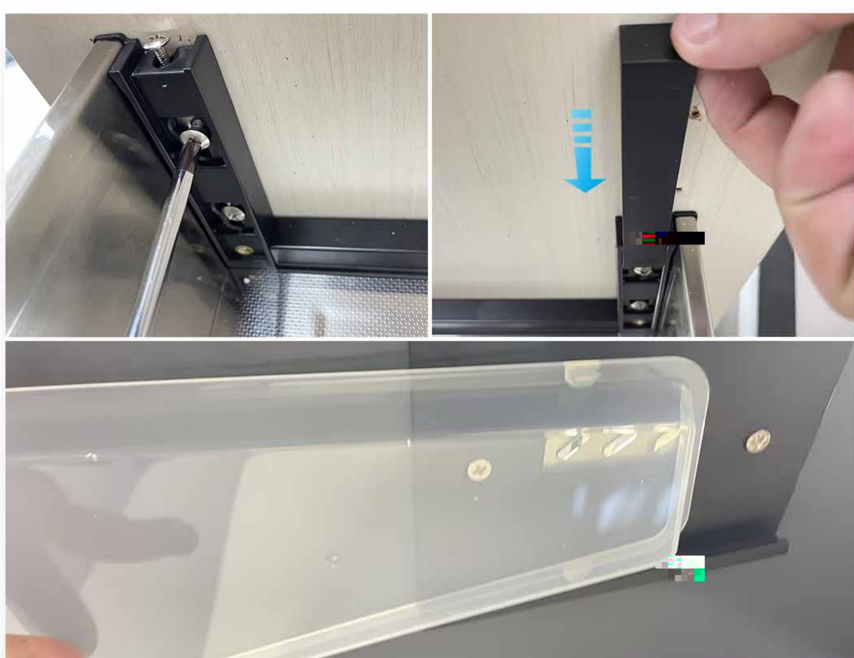
门板与平篮组装，并调整门板，安装装饰盖 挂上接水盘
